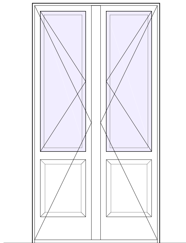
se.2 porta d'ingresso dim. vano luce cm 111x209h superficie mq 2.32 movimento apertura alla francese vetri 3+3/16/3+3 trasparente scuri interni
